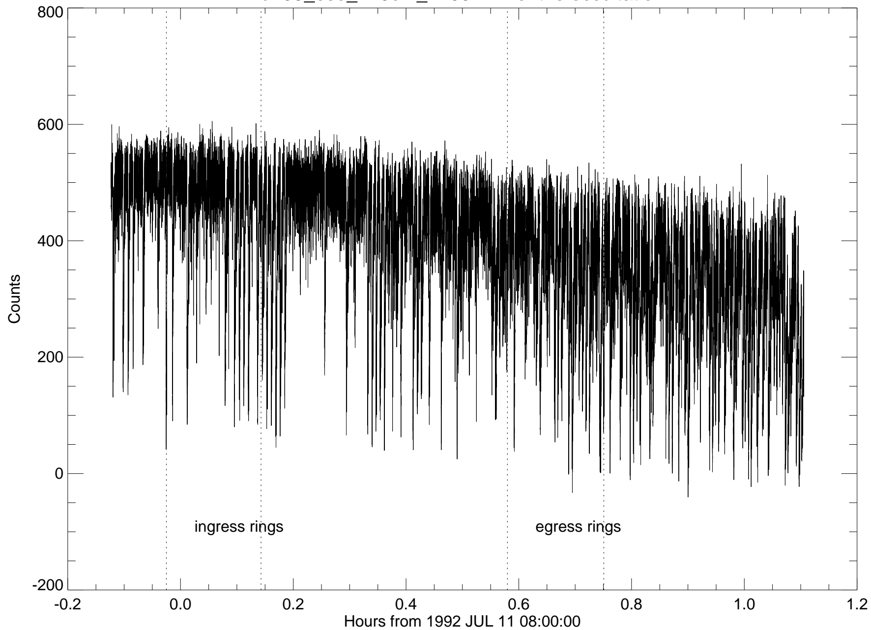
u103_eso_220cm_220nm - entire occultation
