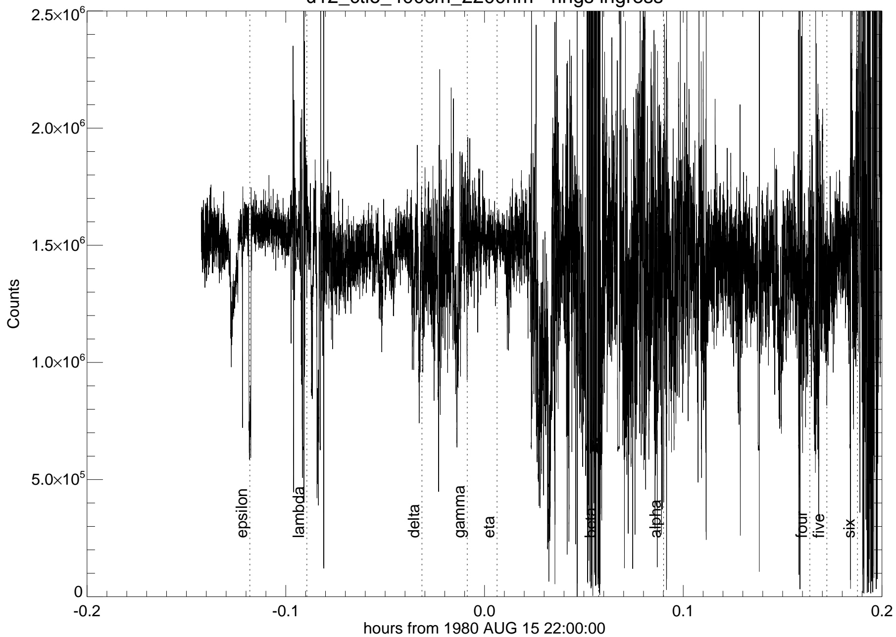
u12_ctio_400cm_2200nm - rings ingress
