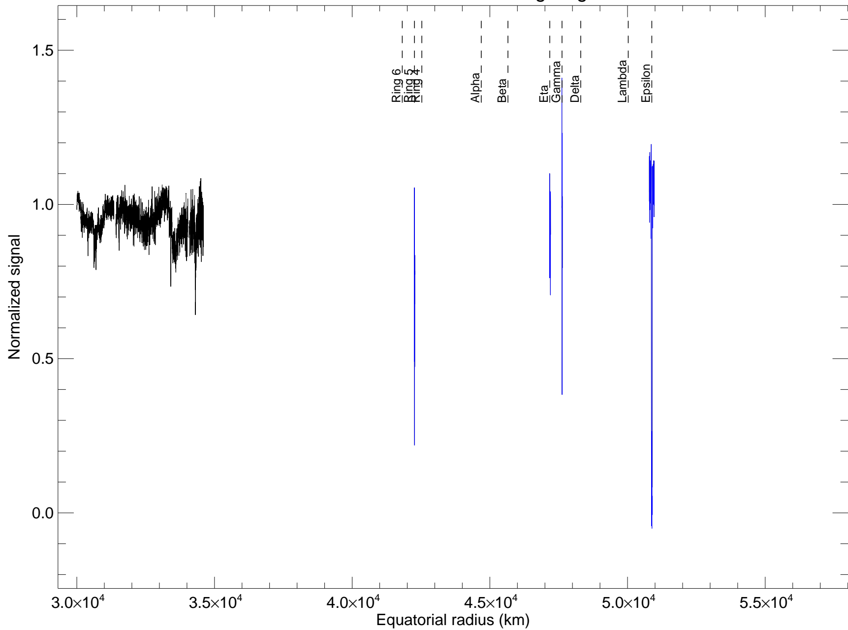
u12_ctio_400cm_2200nm rings ingress
