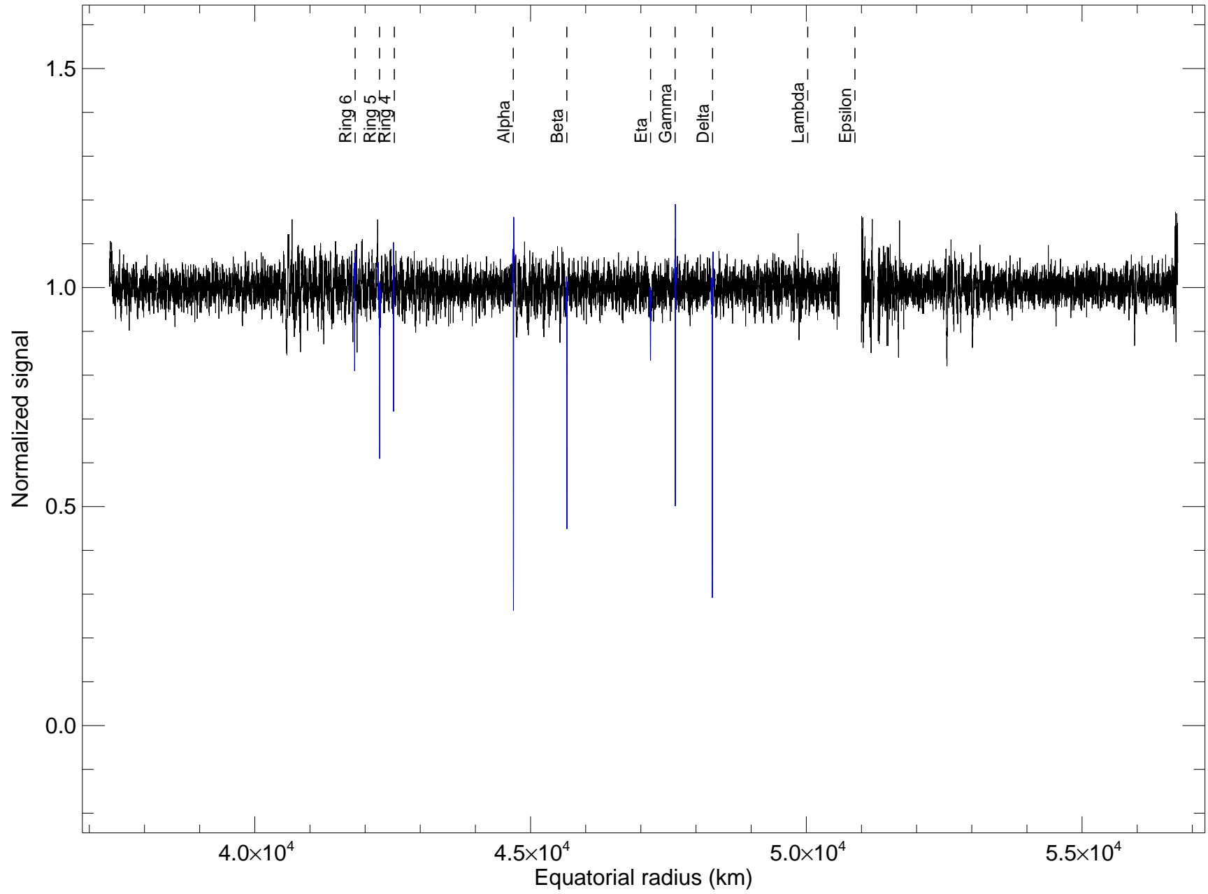
u12_eso_360cm_2200nm rings ingress
