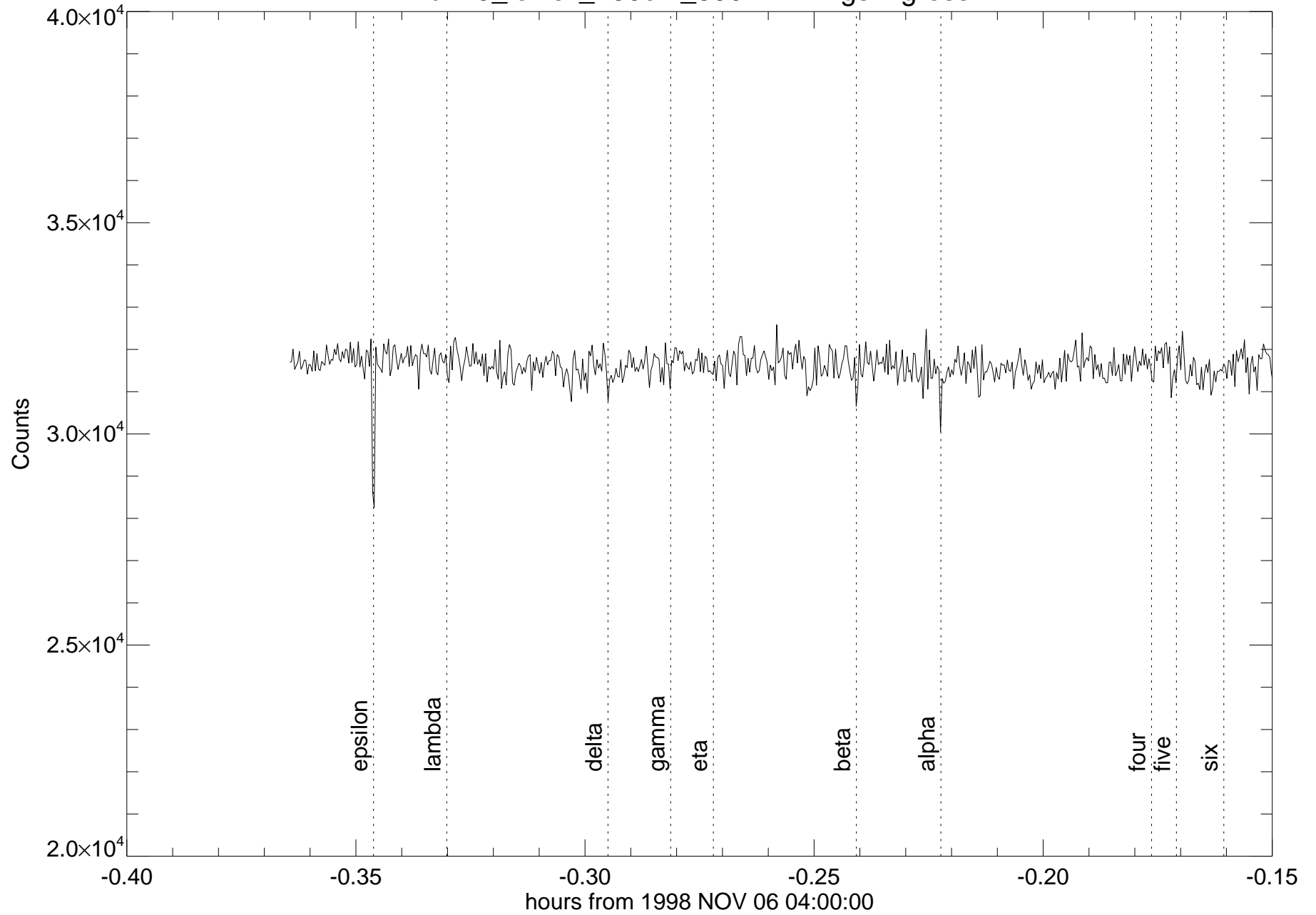
u149_lowell_180cm_890nm - rings ingress
