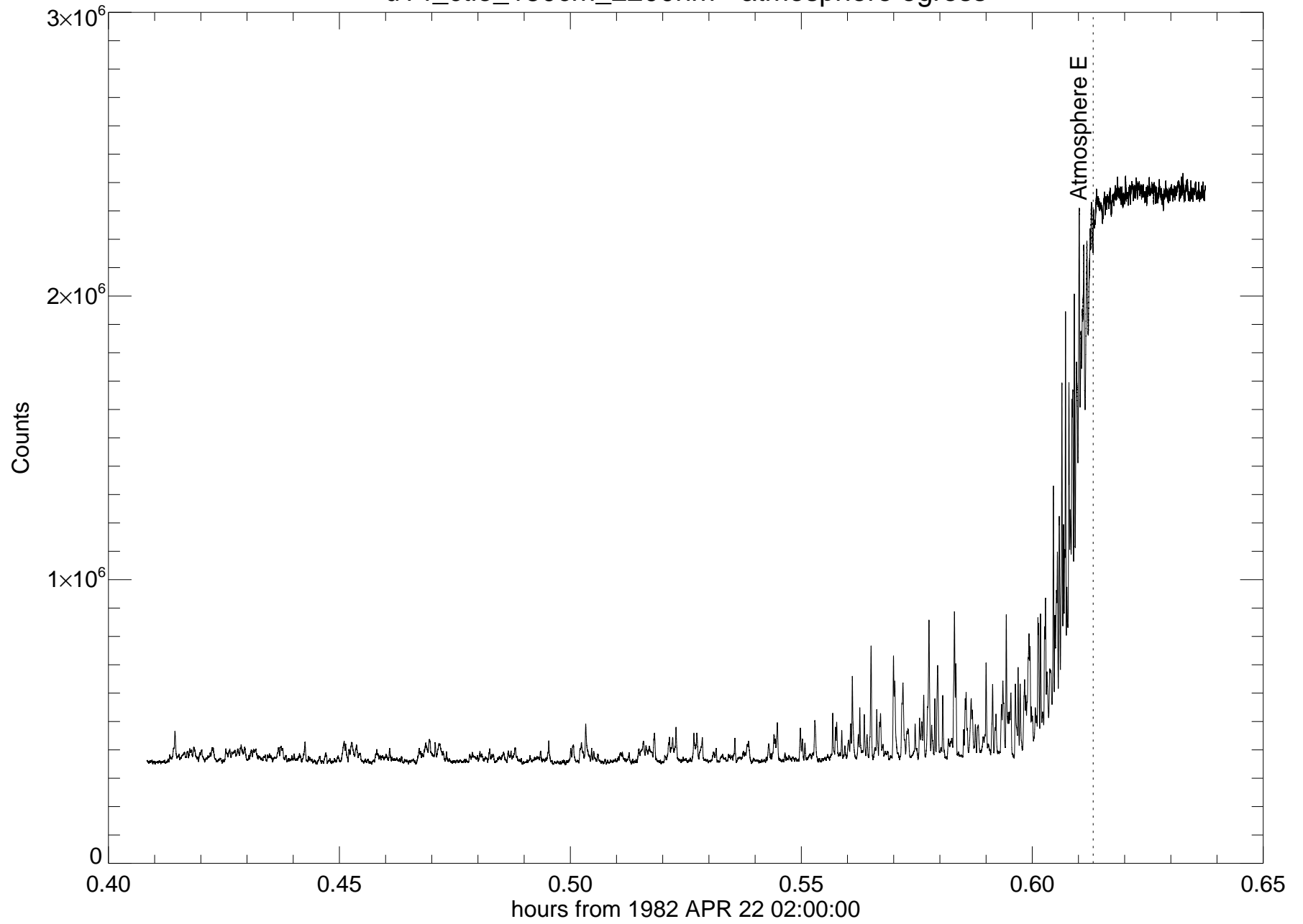
u14_ctio_150cm_2200nm - atmosphere egress
