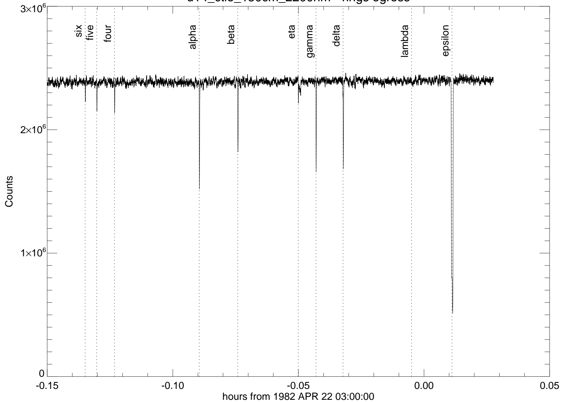
u14_ctio_150cm_2200nm - rings egress
