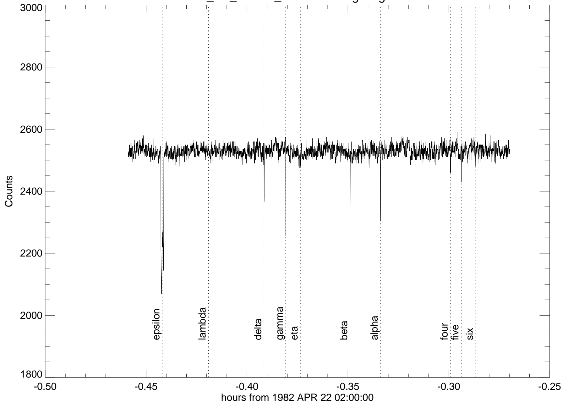
u14_lco_250cm_2200nm - rings ingress
