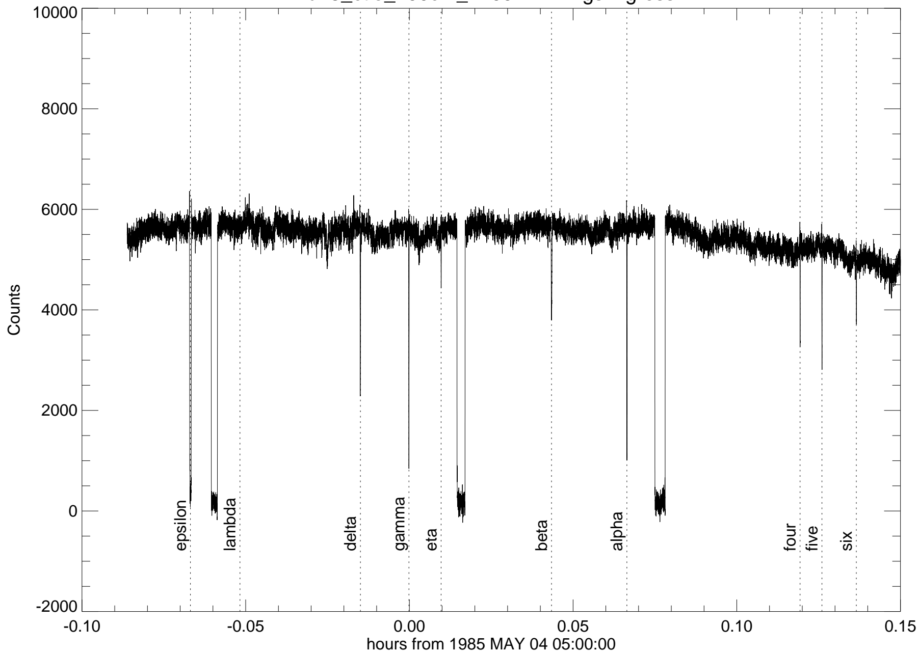
u23_ctio_400cm_2200nm - rings ingress
