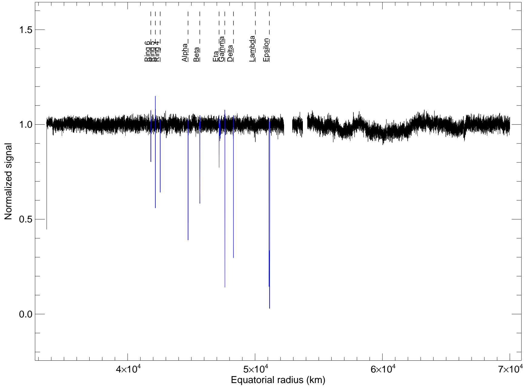
u23_ctio_400cm_2200nm rings egress
