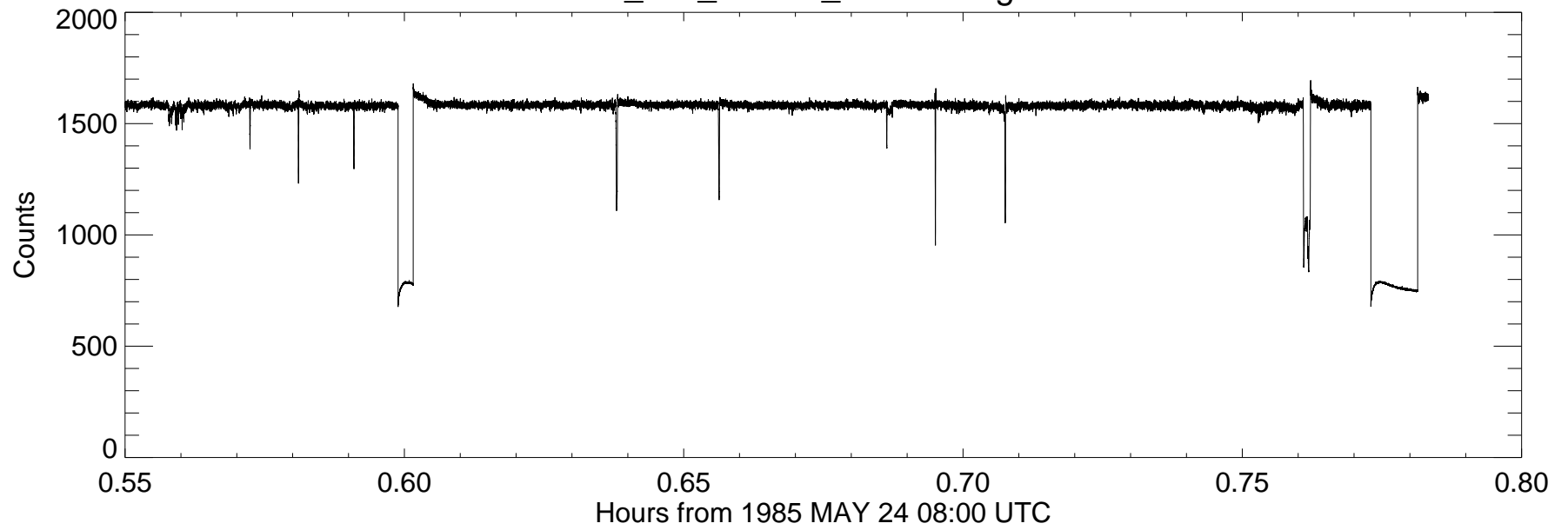
u25_ctio_400cm_2200nm egress
