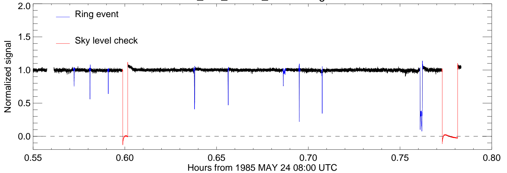
u25_ctio_400cm_2200nm egress
