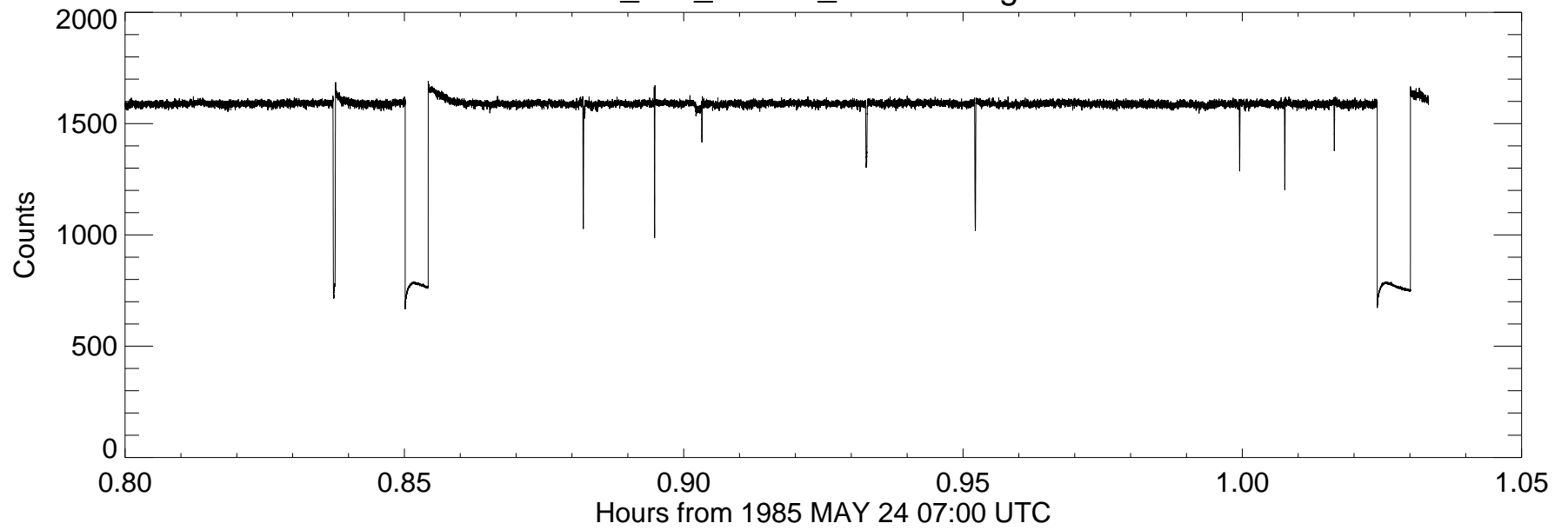
u25_ctio_400cm_2200nm ingress
