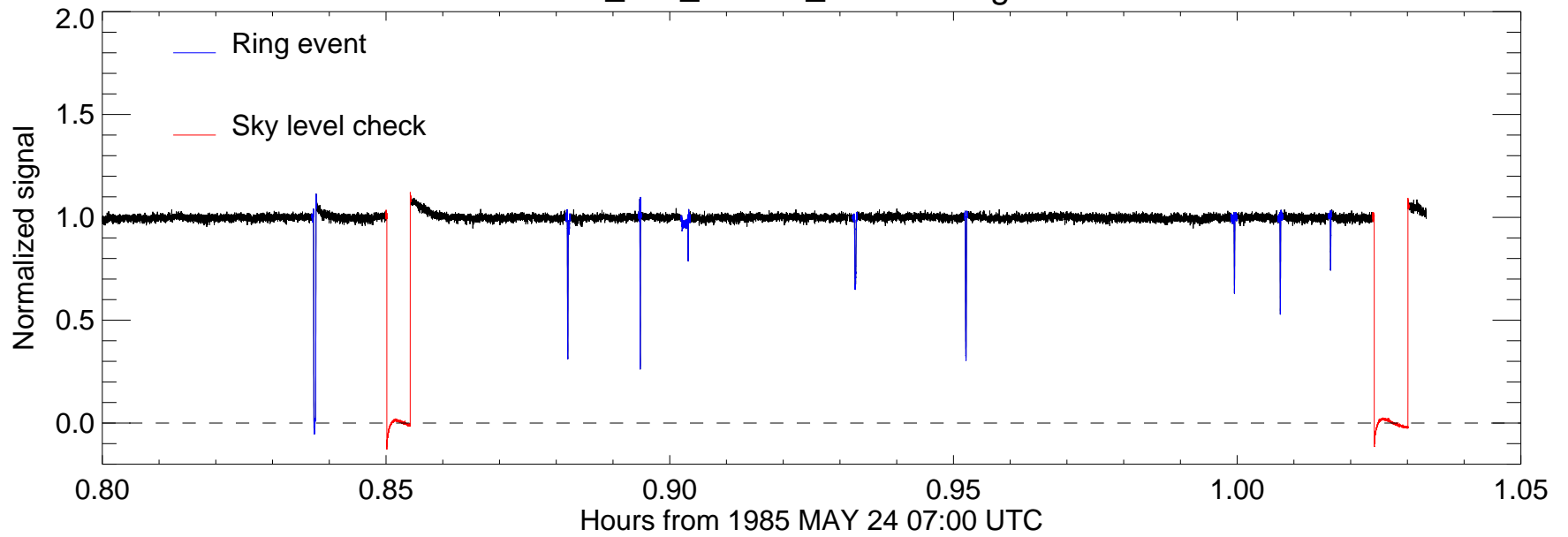
u25_ctio_400cm_2200nm ingress
