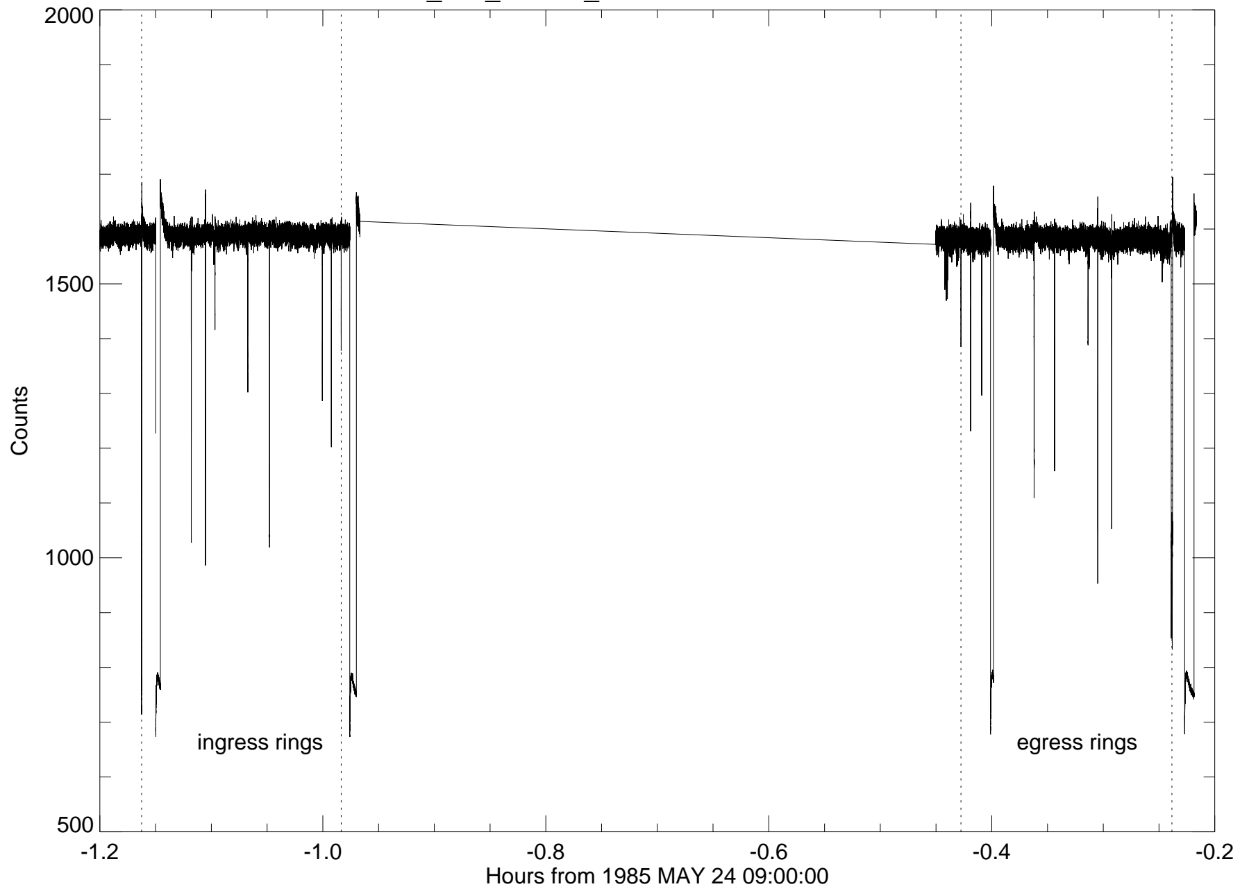
u25_ctio_400cm_2200nm - entire occultation
