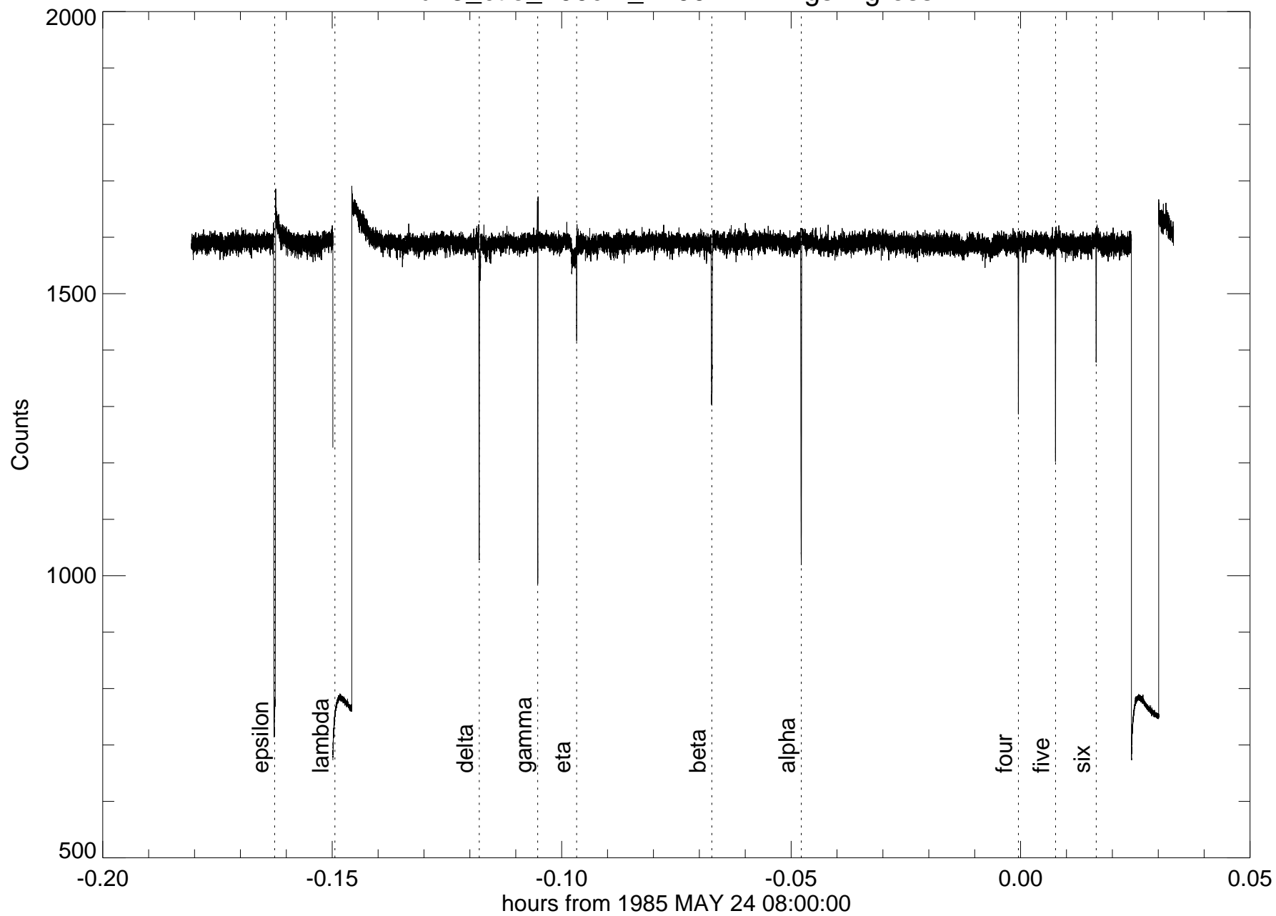
u25_ctio_400cm_2200nm - rings ingress
