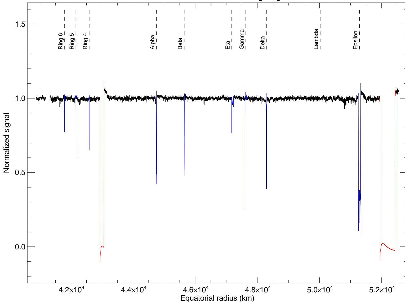
u25_ctio_400cm_2200nm rings egress
