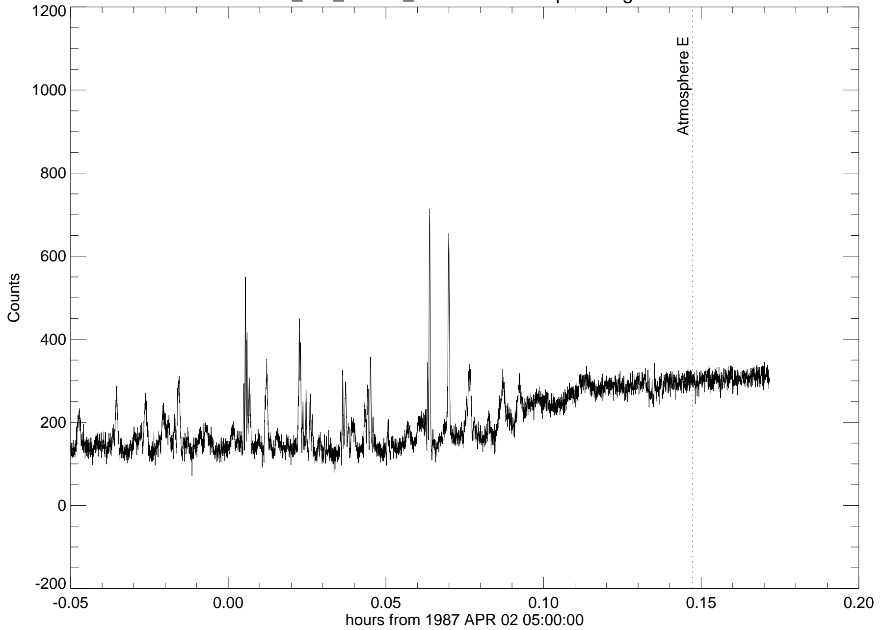
u36_ctio_400cm_2200nm - atmosphere egress
