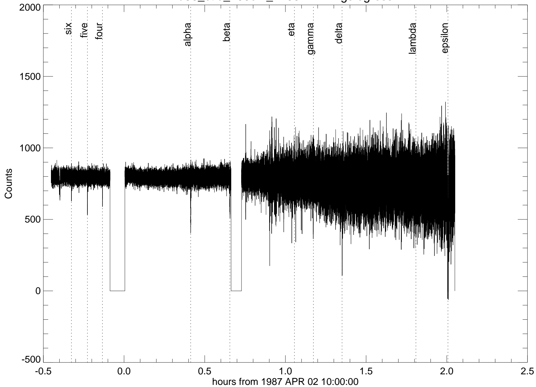
u36_ctio_400cm_2200nm - rings egress
