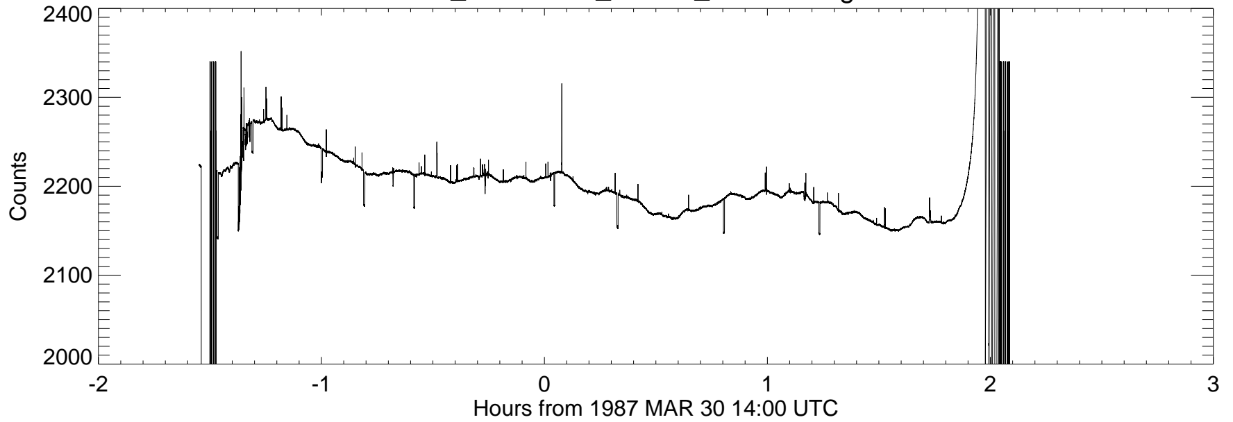
u36_maunakea_380cm_2200nm ingress
