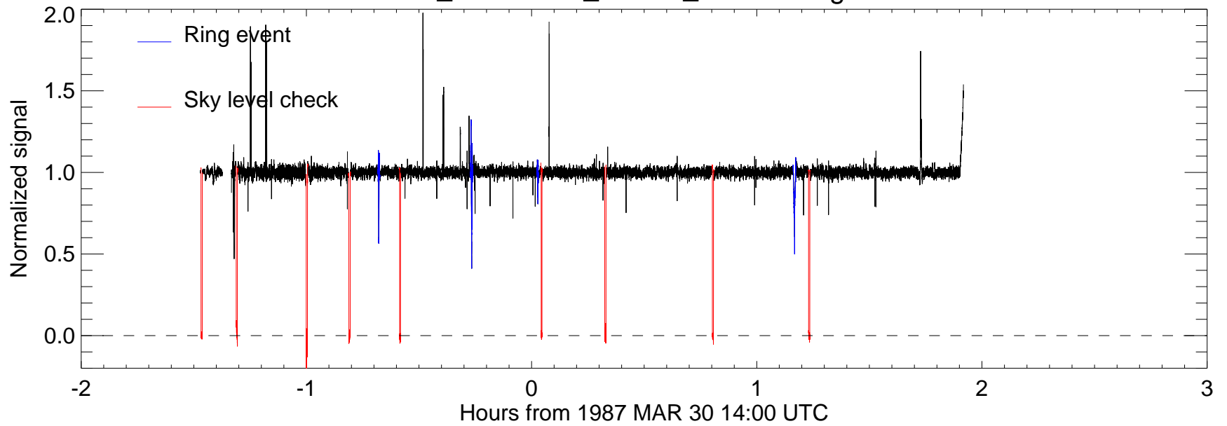
u36_maunakea_380cm_2200nm ingress
