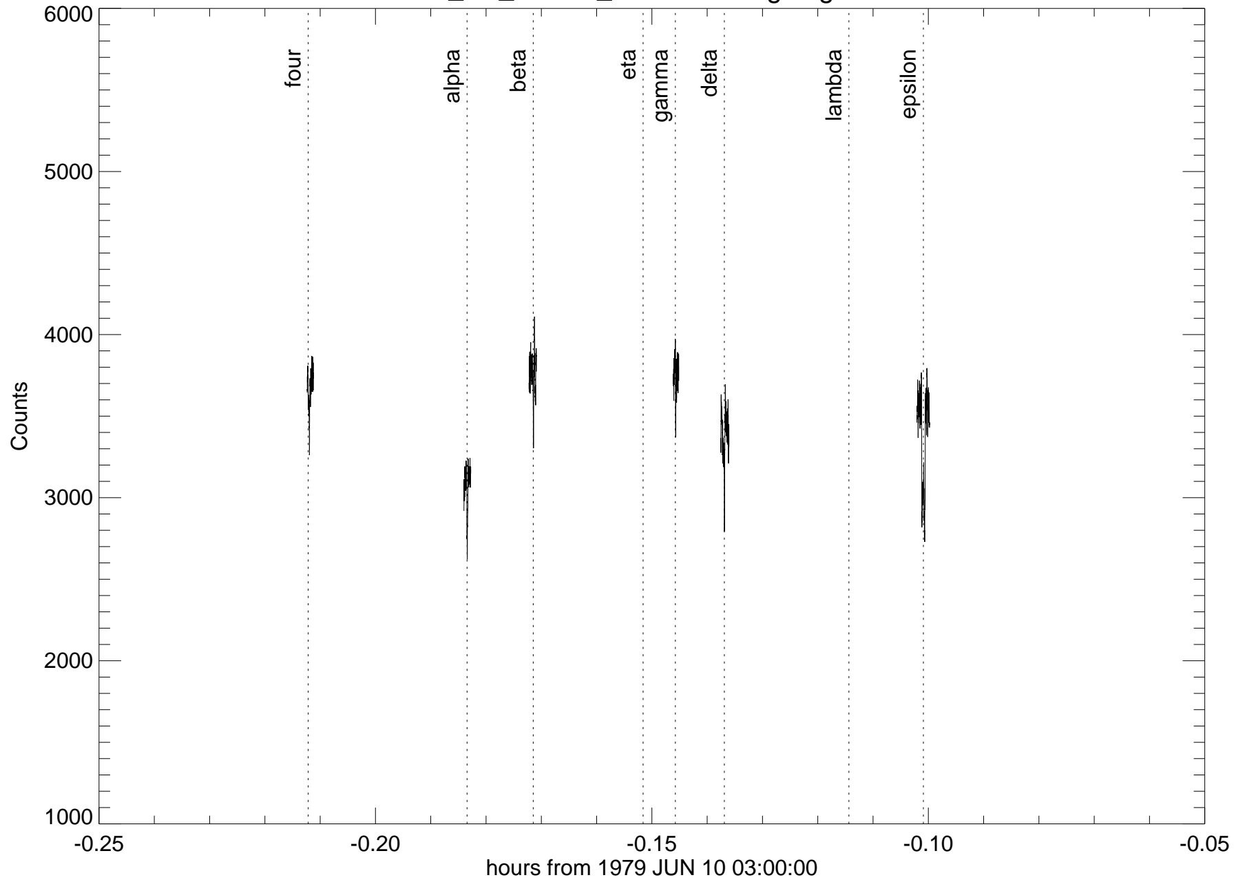
u9_lco_250cm_2200nm - rings egress
