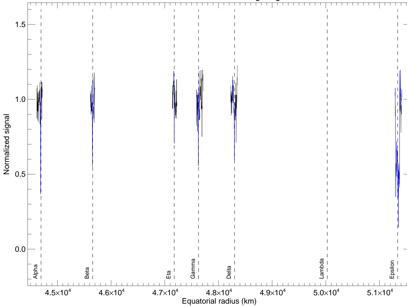
u9_lco_250cm_2200nm rings ingress
