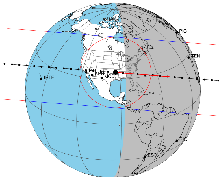
2033-03-29T23:56:08.2800 α: 06 02 01.7537 δ: +22 44 43.028 C/A 0.199" PA 4.50 deg v_sky + 8.99 km/s D 09.11 AU
