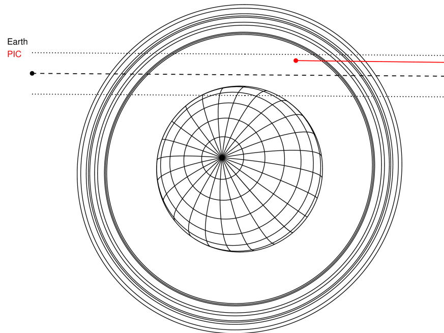
Uranus 2032-08-12T01:24:55 K14.40 G17.62 PRgt
