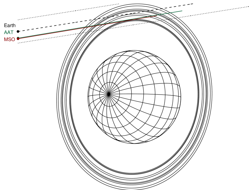
Uranus 2038-05-11T10:23:02 K14.65 G18.68 XRgt
